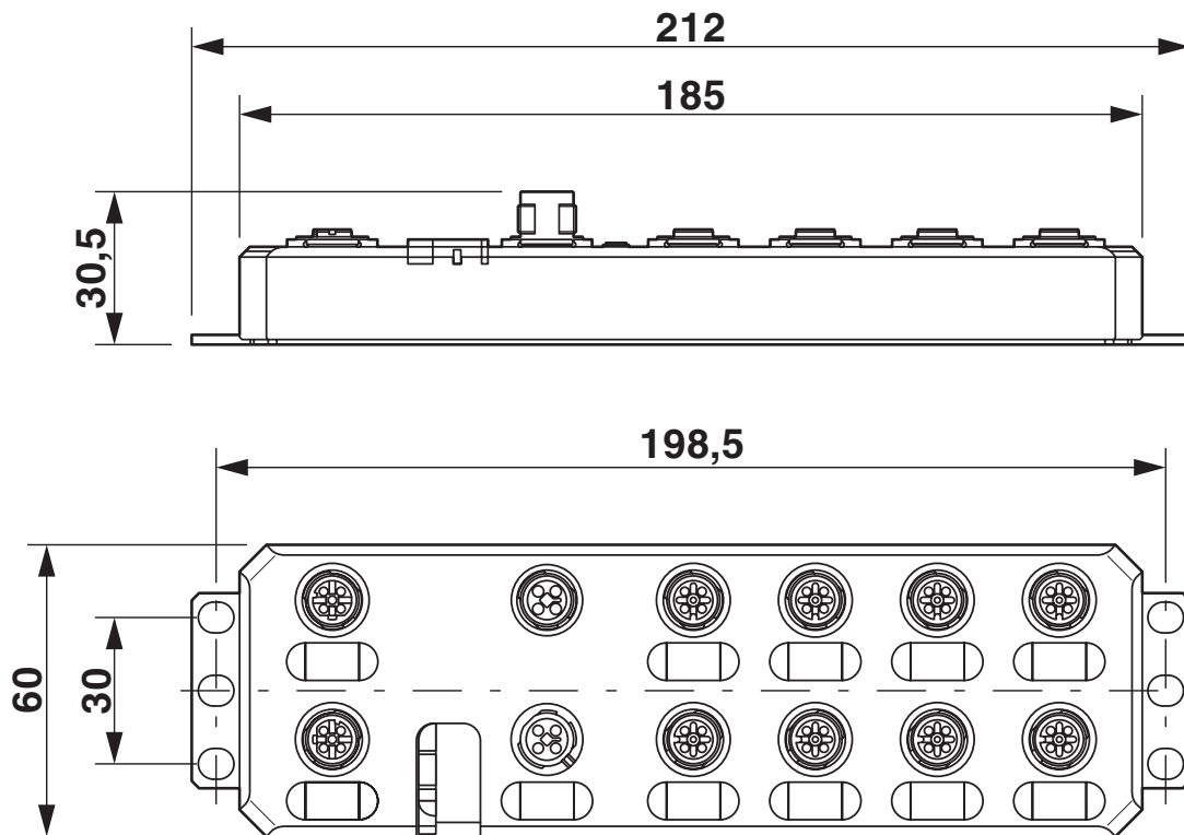
Rysunek wymiarowy
