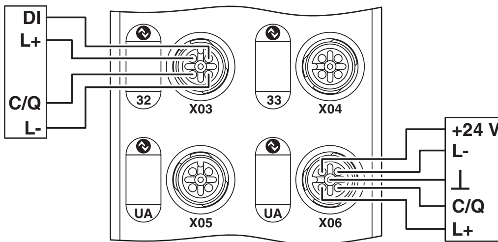
rysunek złączy
