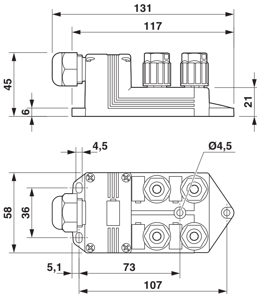
Rysunek wymiarowy
