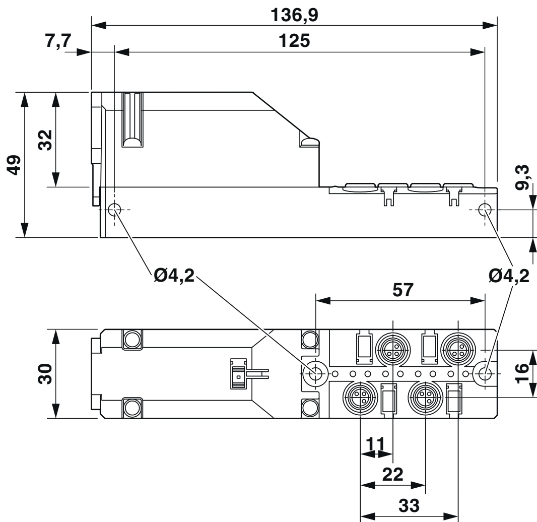
Rysunek wymiarowy
