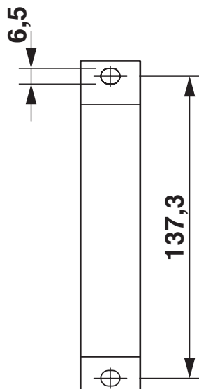
Rysunek wymiarowy
