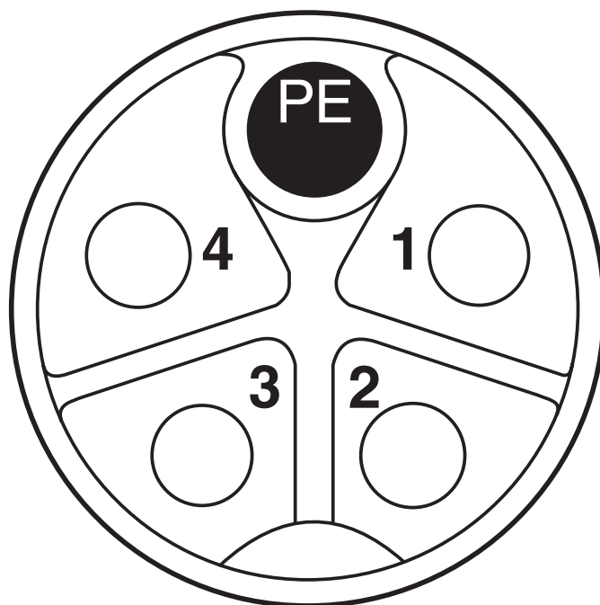
Układ styków gniazda M12, 4-bieg.+PE, kodowanie K, widok złącza żeńskiego
