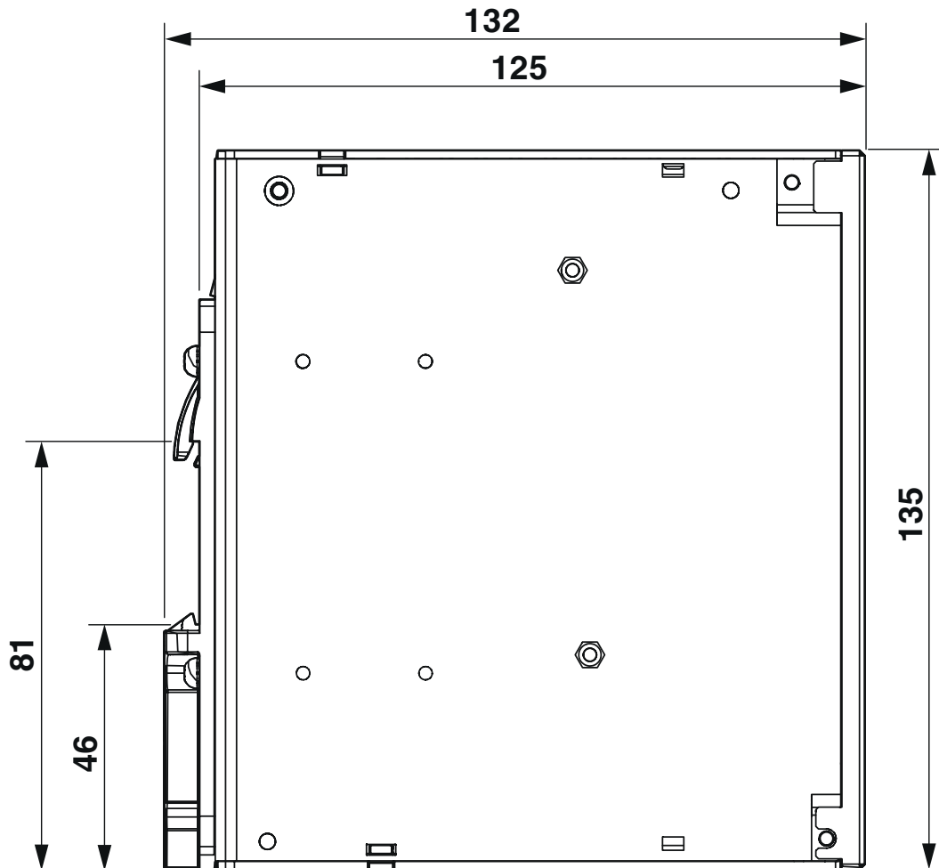
Rysunek wymiarowy
