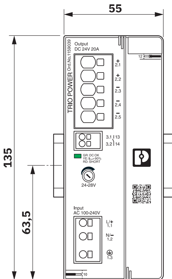
Rysunek wymiarowy
