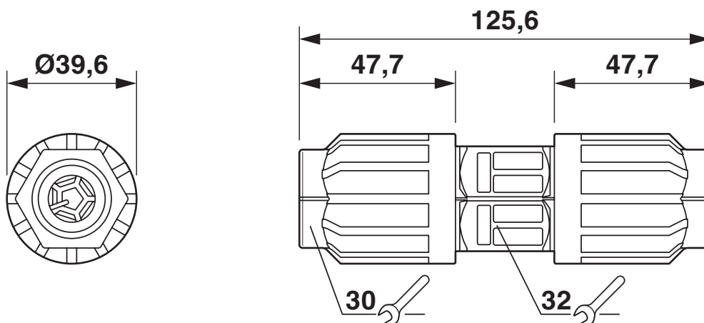
Rysunek wymiarowy QPD C 5x6,0
