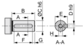
DIN 6885 A
