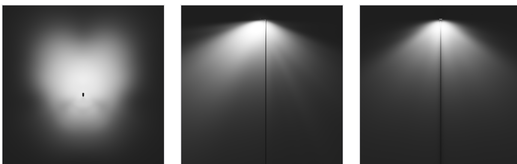
Rozsył na przejścia dla pieszych PC (ang. Pedestrian Crossing)
