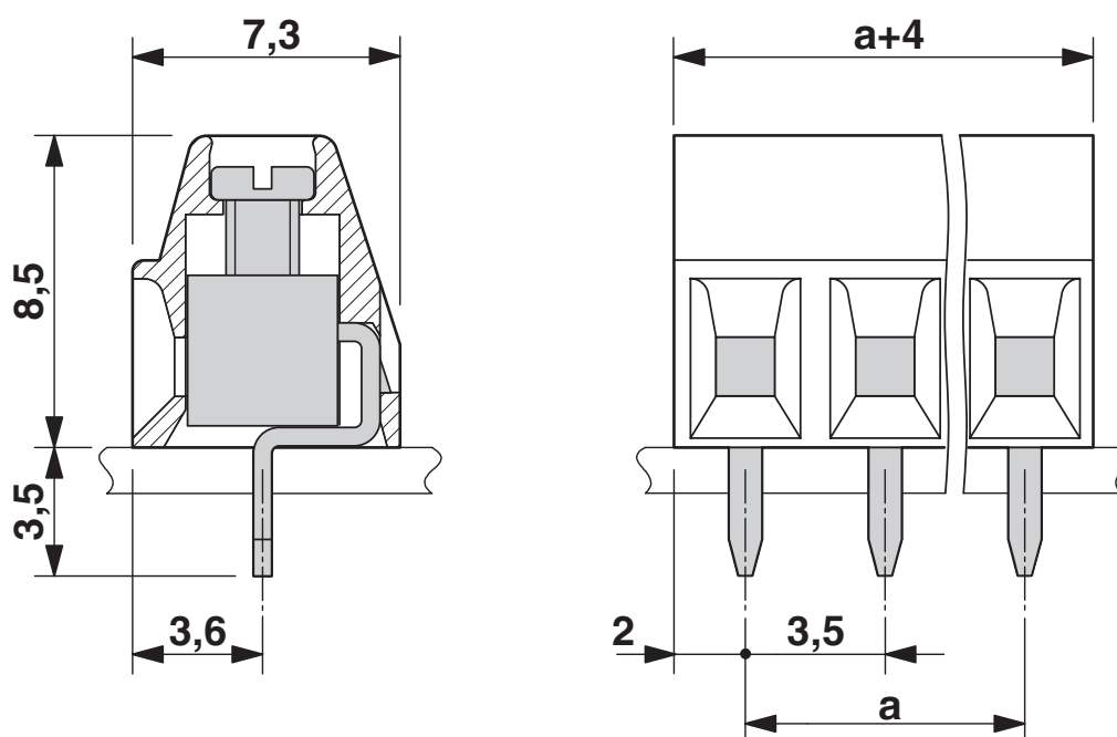
Rysunek wymiarowy
