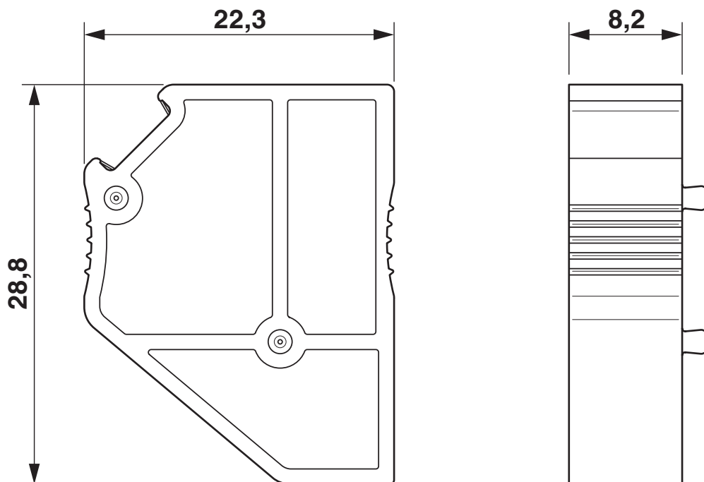
Rysunek wymiarowy
