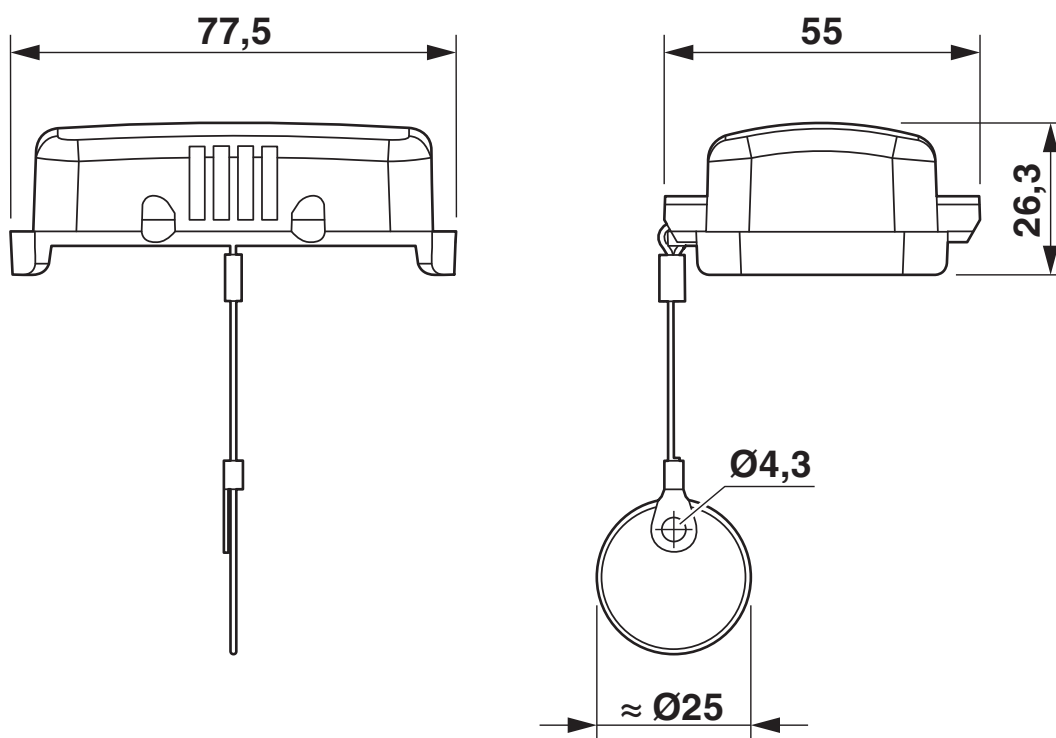
Rysunek wymiarowy
