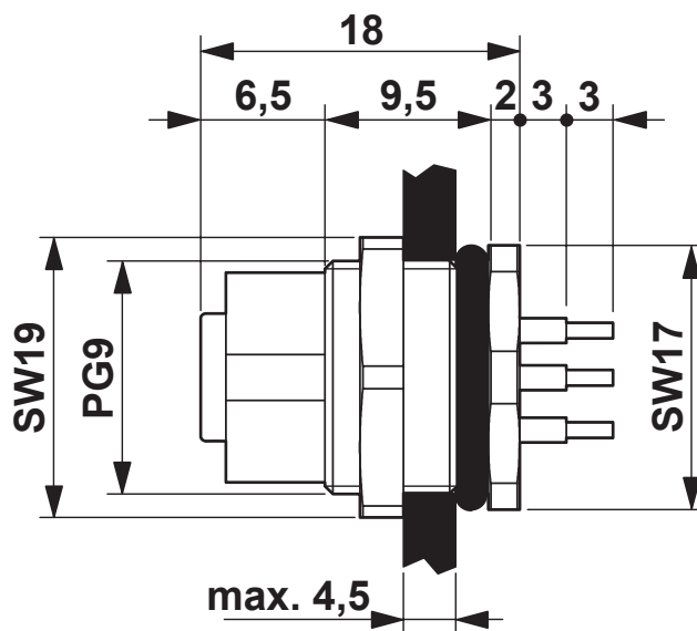
Rysunek wymiarowy
