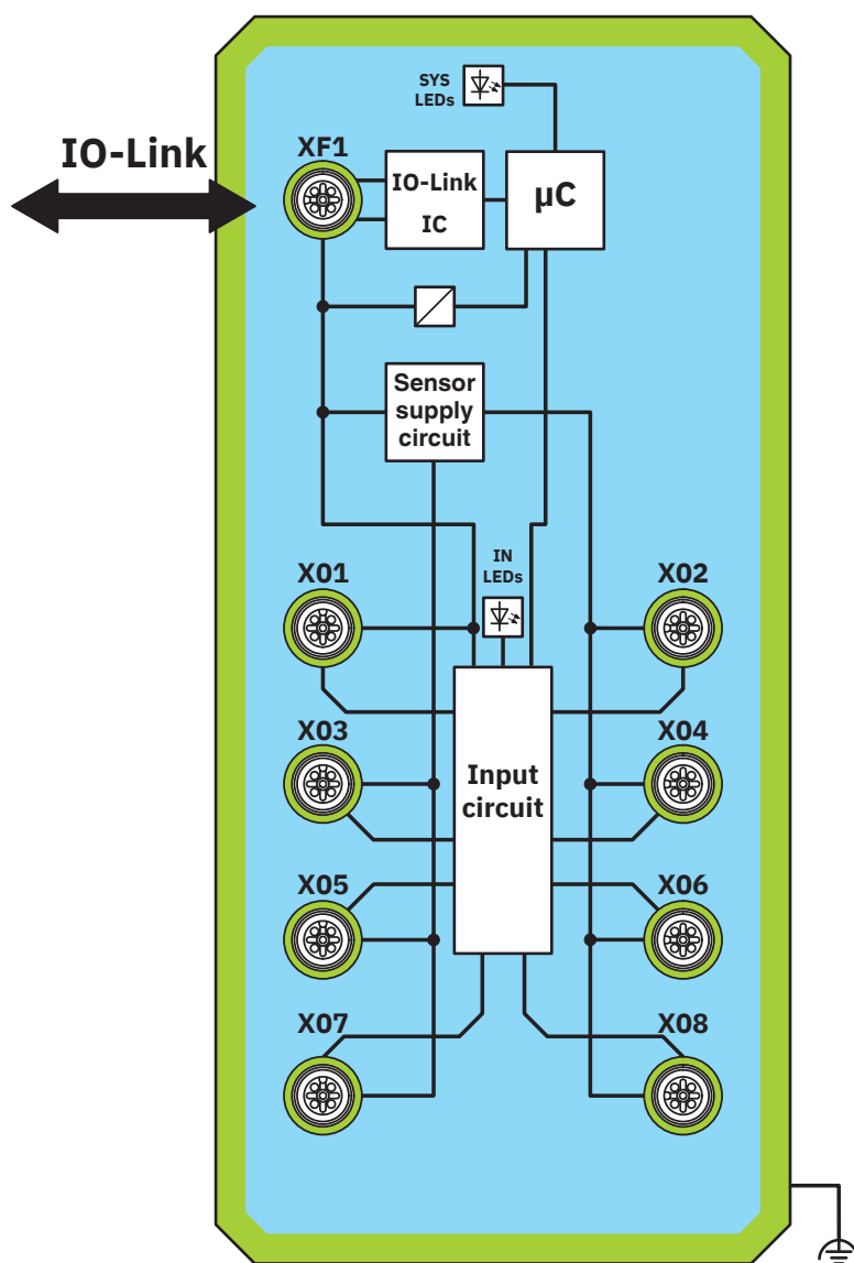
Schemat blokowy
