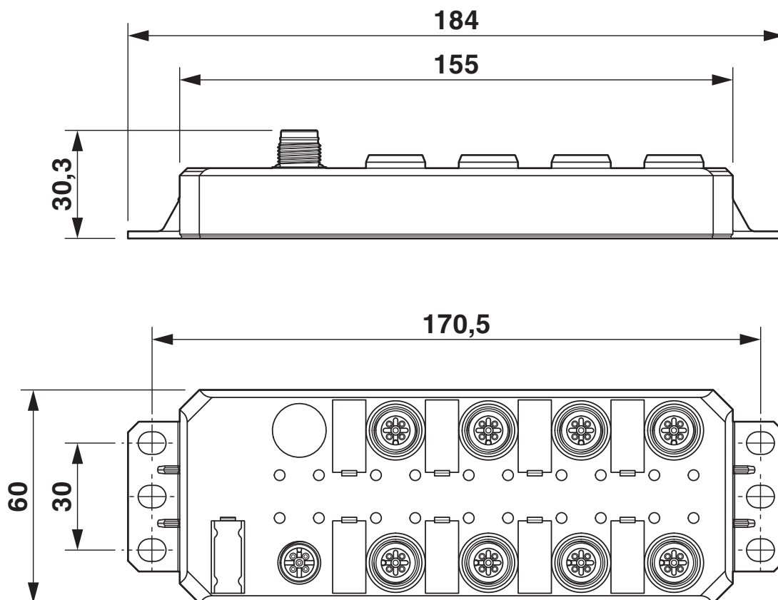
Rysunek wymiarowy
