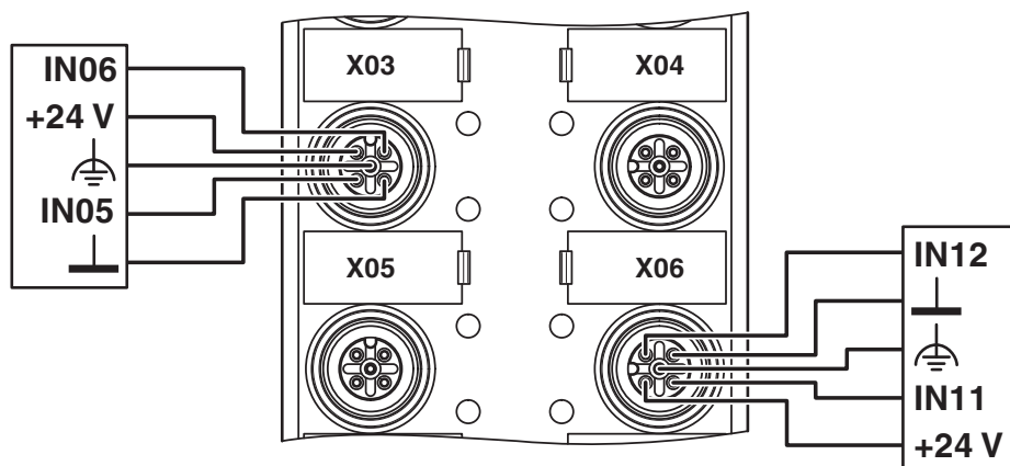
rysunek złączy
