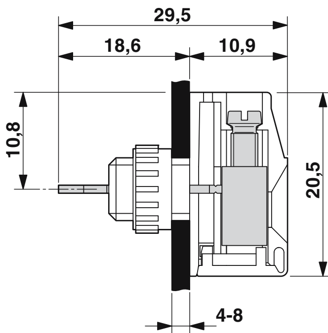
Rysunek wymiarowy
