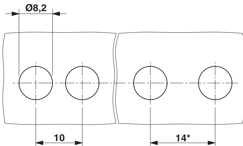
Rysunek wymiarowy
