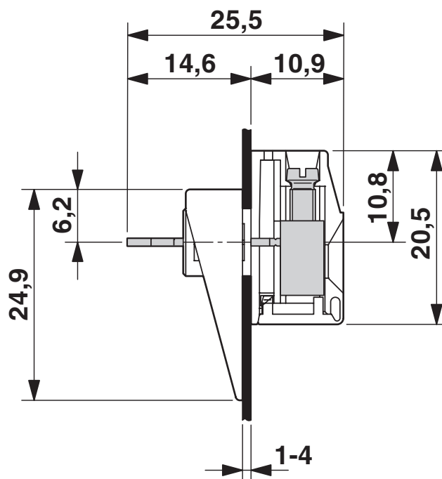
Rysunek wymiarowy
