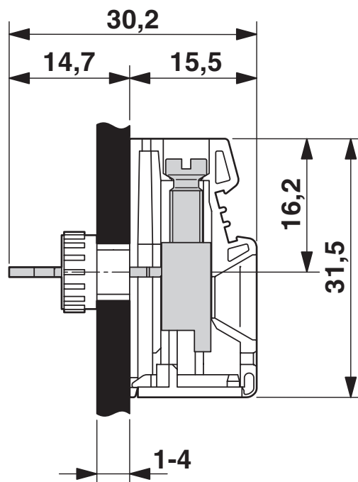
Rysunek wymiarowy
