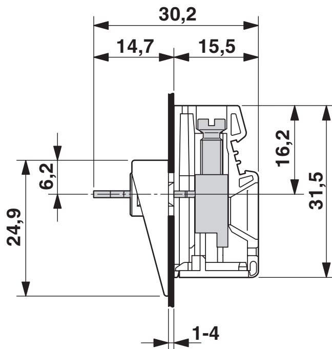
Rysunek wymiarowy
