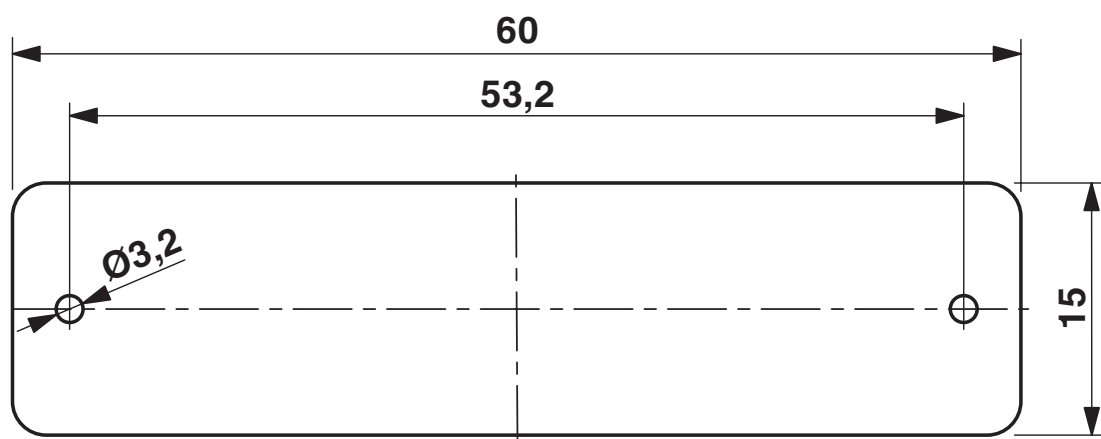
Rysunek wymiarowy
