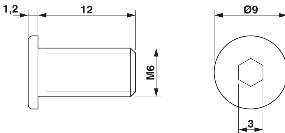
Rysunek wymiarowy
