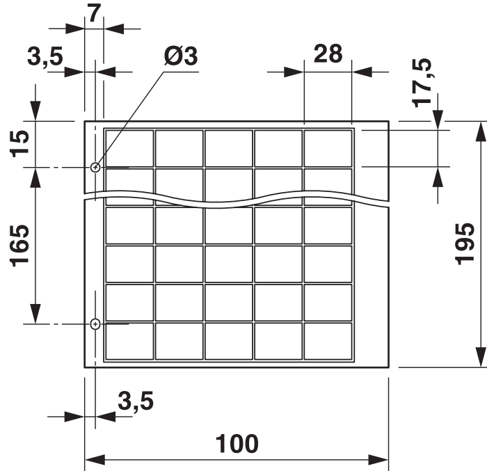
Rysunek wymiarowy
