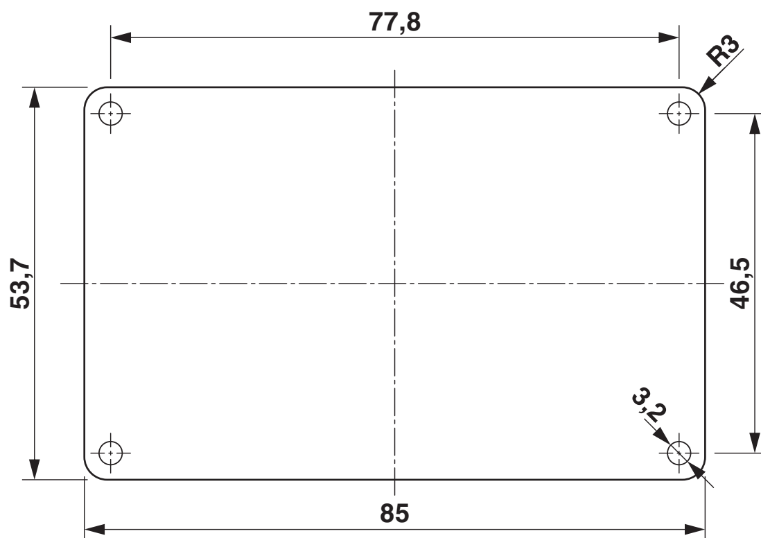
Rysunek wymiarowy
