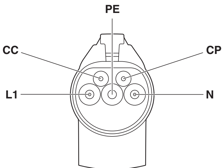
Rysunek schematyczny
