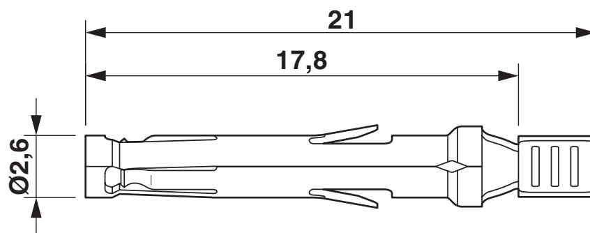
Rysunek wymiarowy
