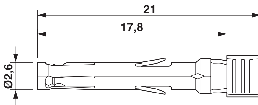
Rysunek wymiarowy
