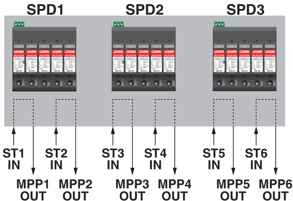
rysunek złączy
