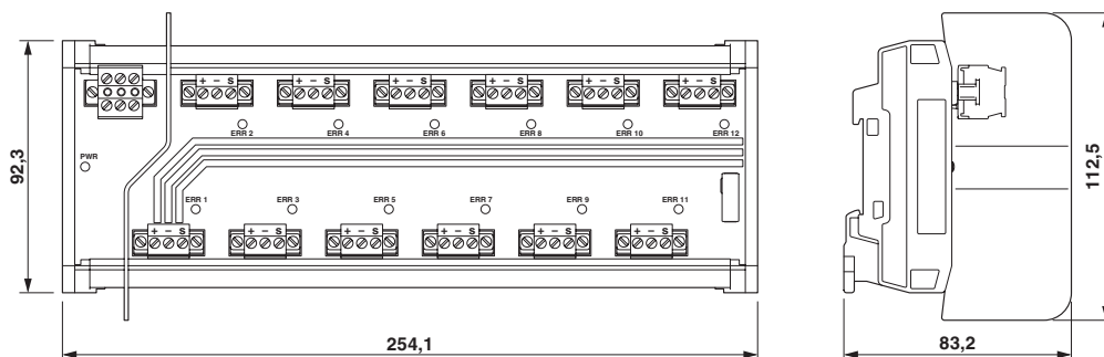
Rysunek wymiarowy
