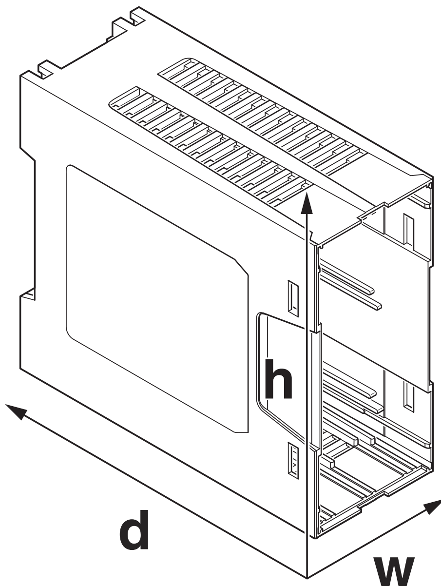
Rysunek wymiarowy
