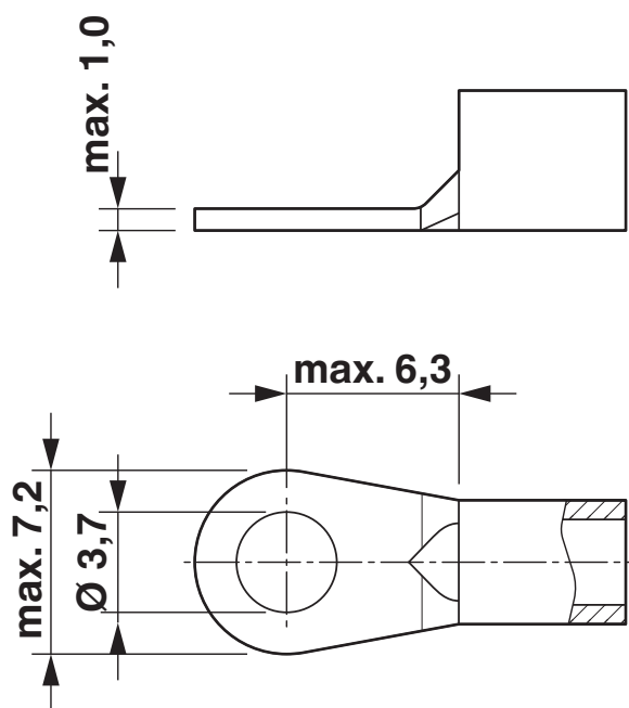
Rysunek wymiarowy
