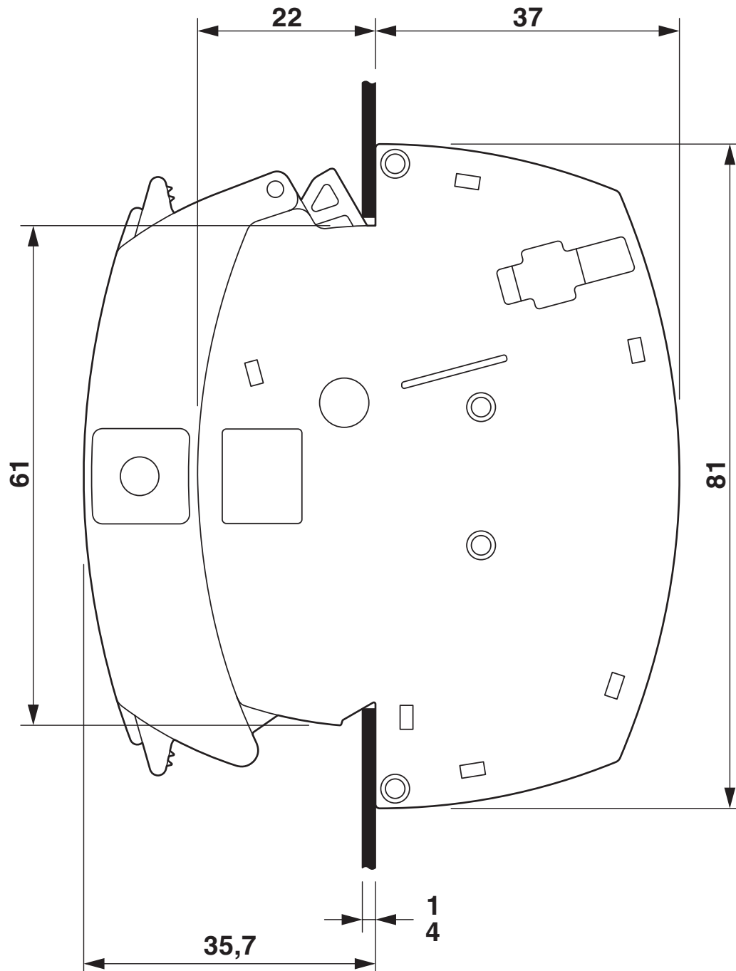
Rysunek wymiarowy
