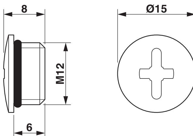
Rysunek wymiarowy
