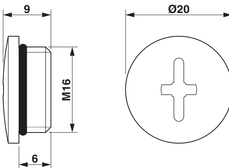
Rysunek wymiarowy
