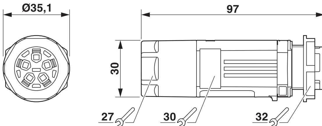
Rysunek wymiarowy
