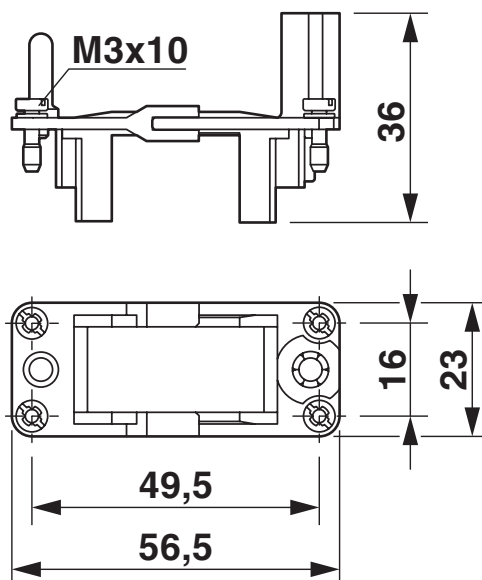
Rysunek wymiarowy
