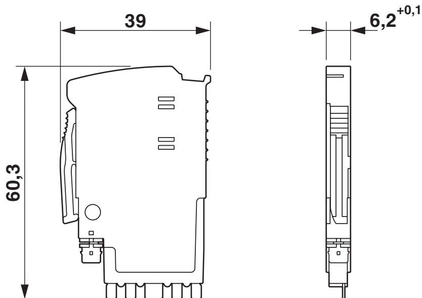
Rysunek wymiarowy
