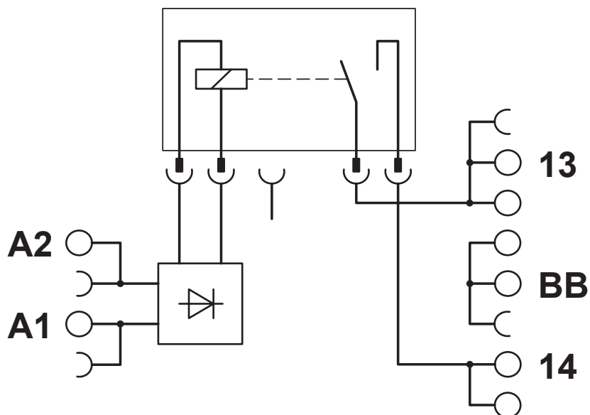
Schemat
