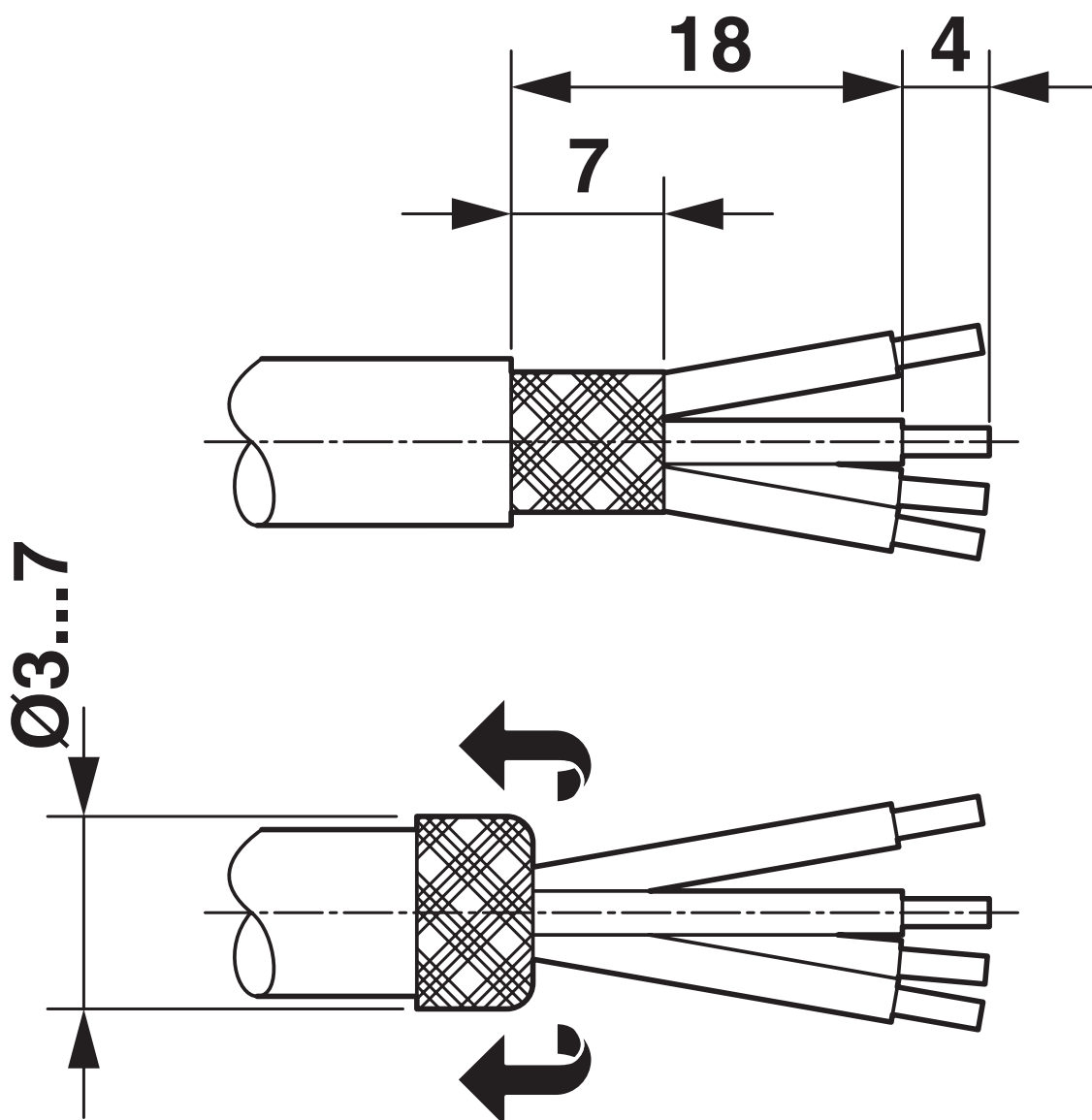
Rysunek wymiarowy
