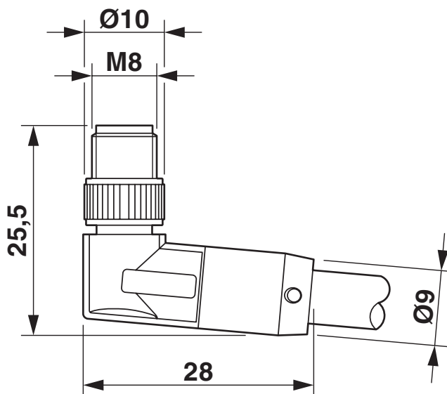
Rysunek wymiarowy
