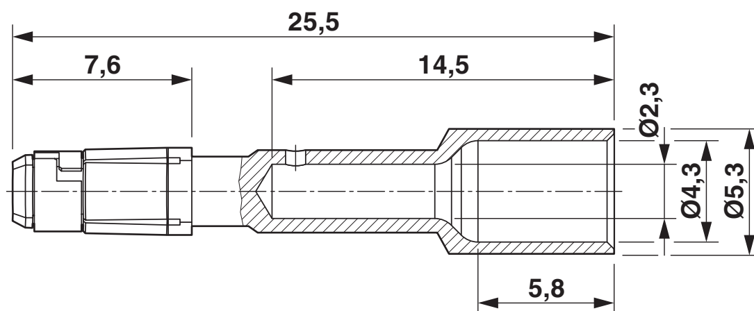
Rysunek wymiarowy
