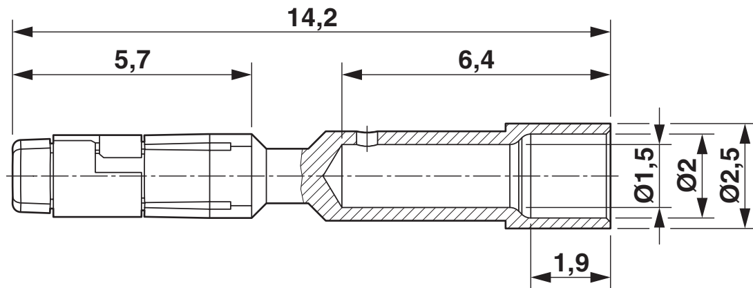
Rysunek wymiarowy
