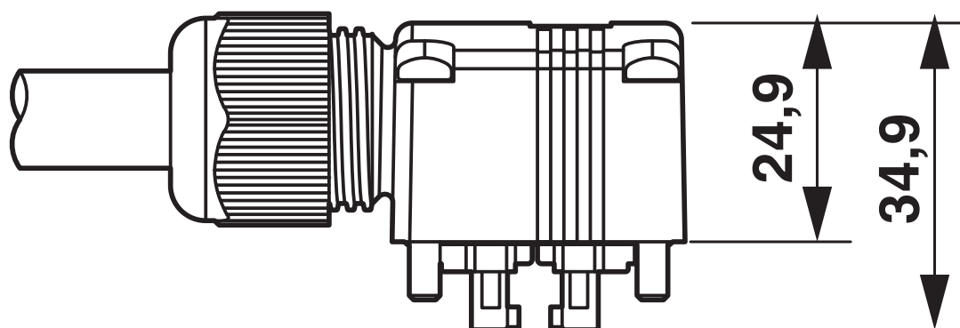
Rysunek wymiarowy
