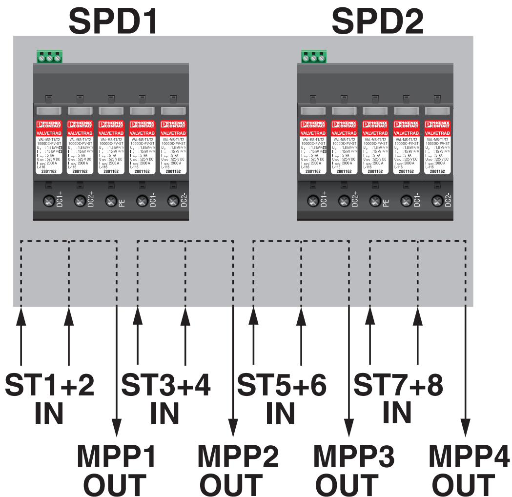
rysunek złączy
