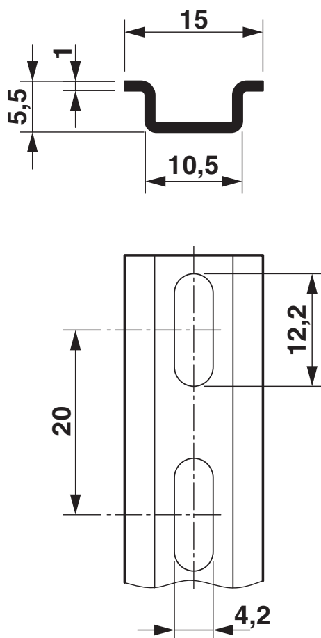
Rysunek wymiarowy
