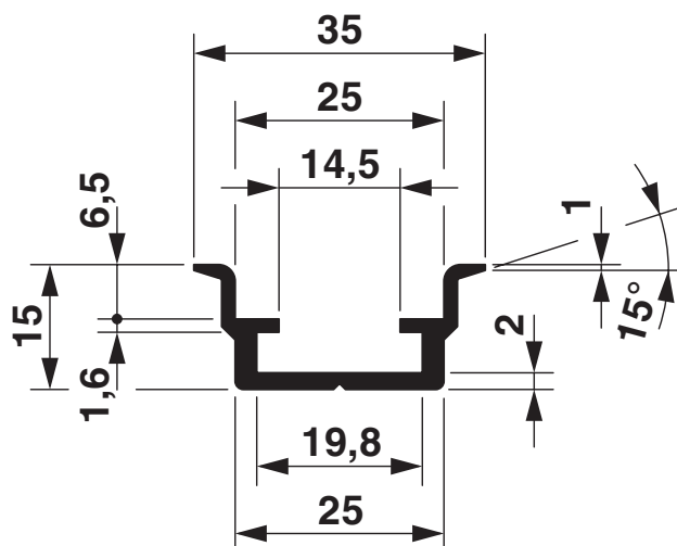
Rysunek wymiarowy
