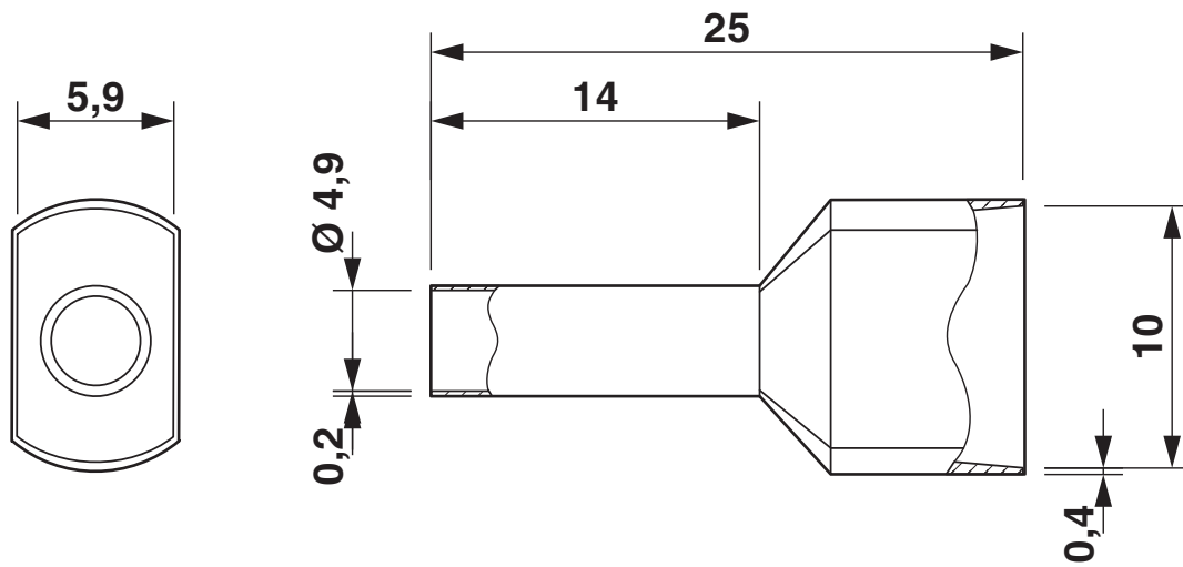
Rysunek wymiarowy
