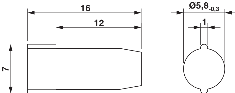
Rysunek wymiarowy
