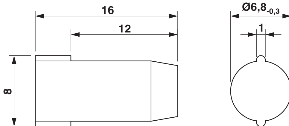
Rysunek wymiarowy
