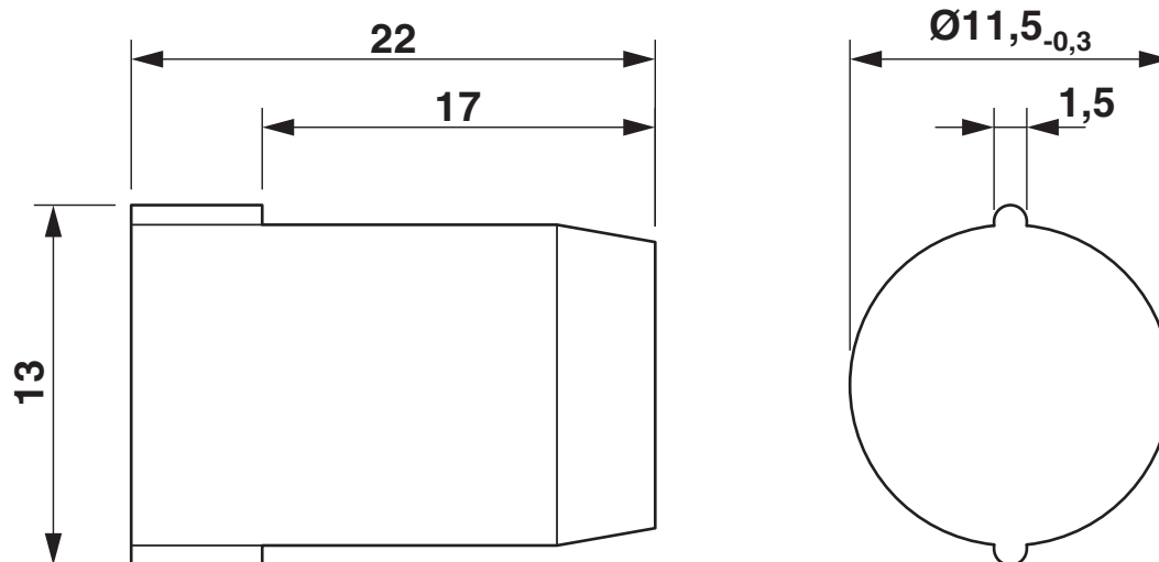
Rysunek wymiarowy
