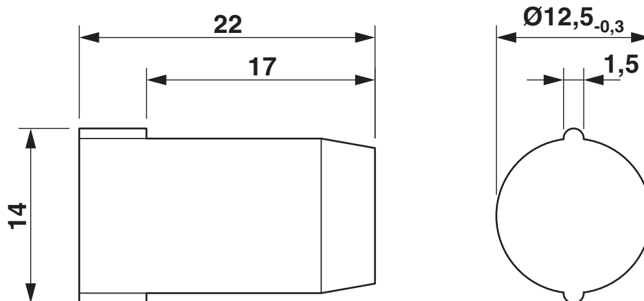
Rysunek wymiarowy
