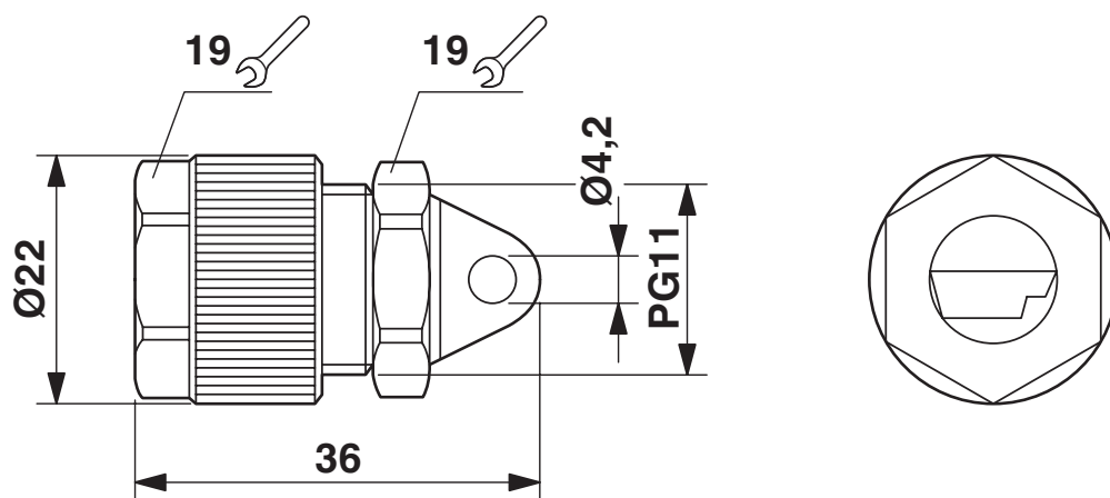
Rysunek wymiarowy
